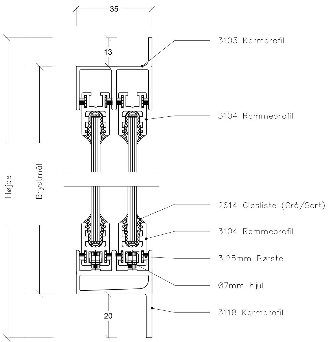
LODRET SNIT 1:1
