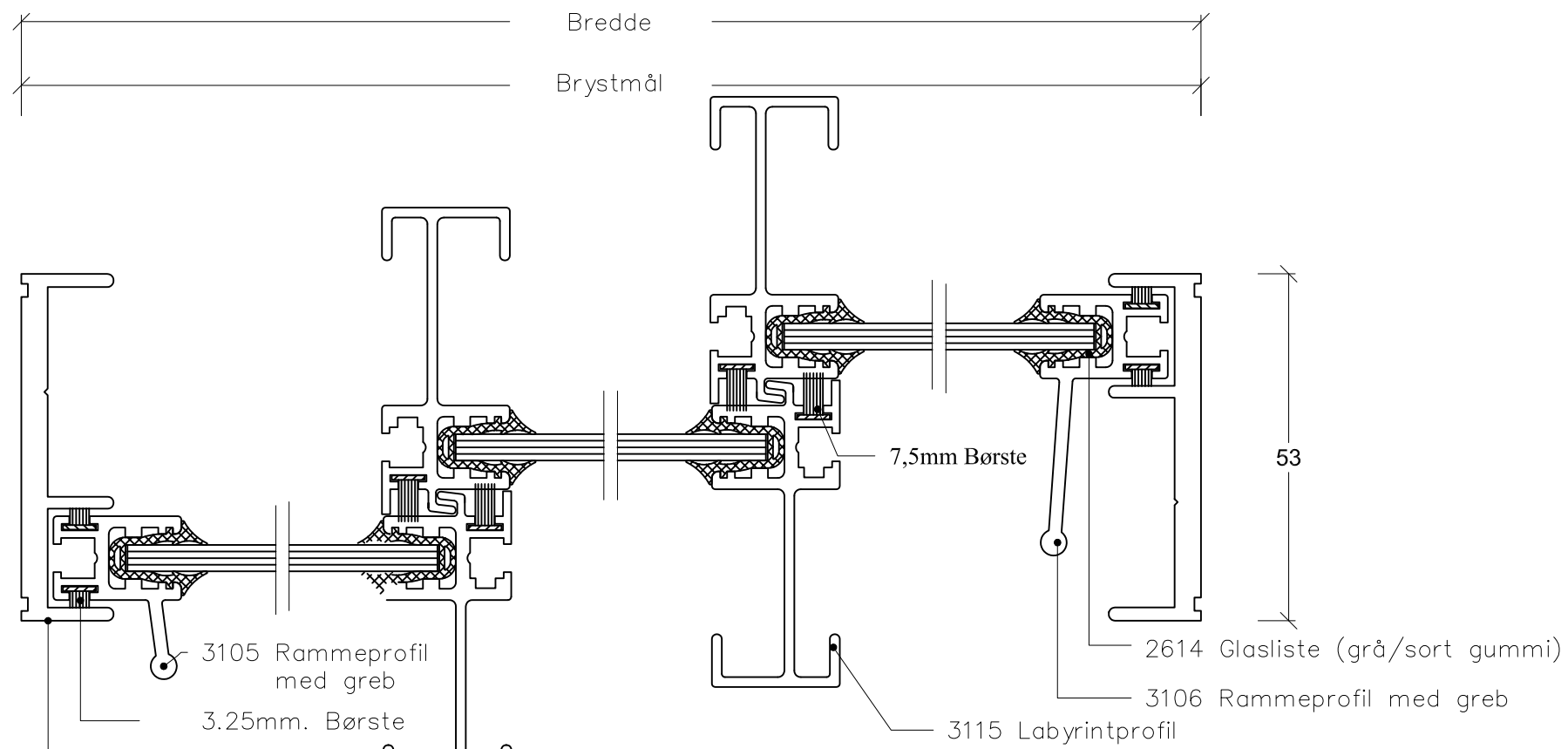
VANDRET SNIT 1:1
