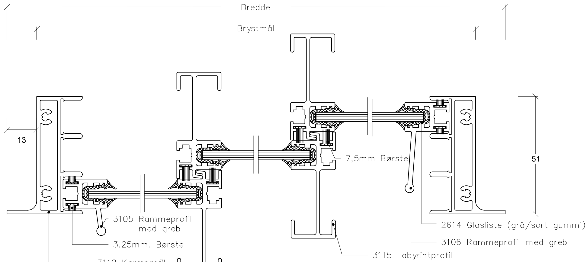
VANDRET SNIT 1:1
