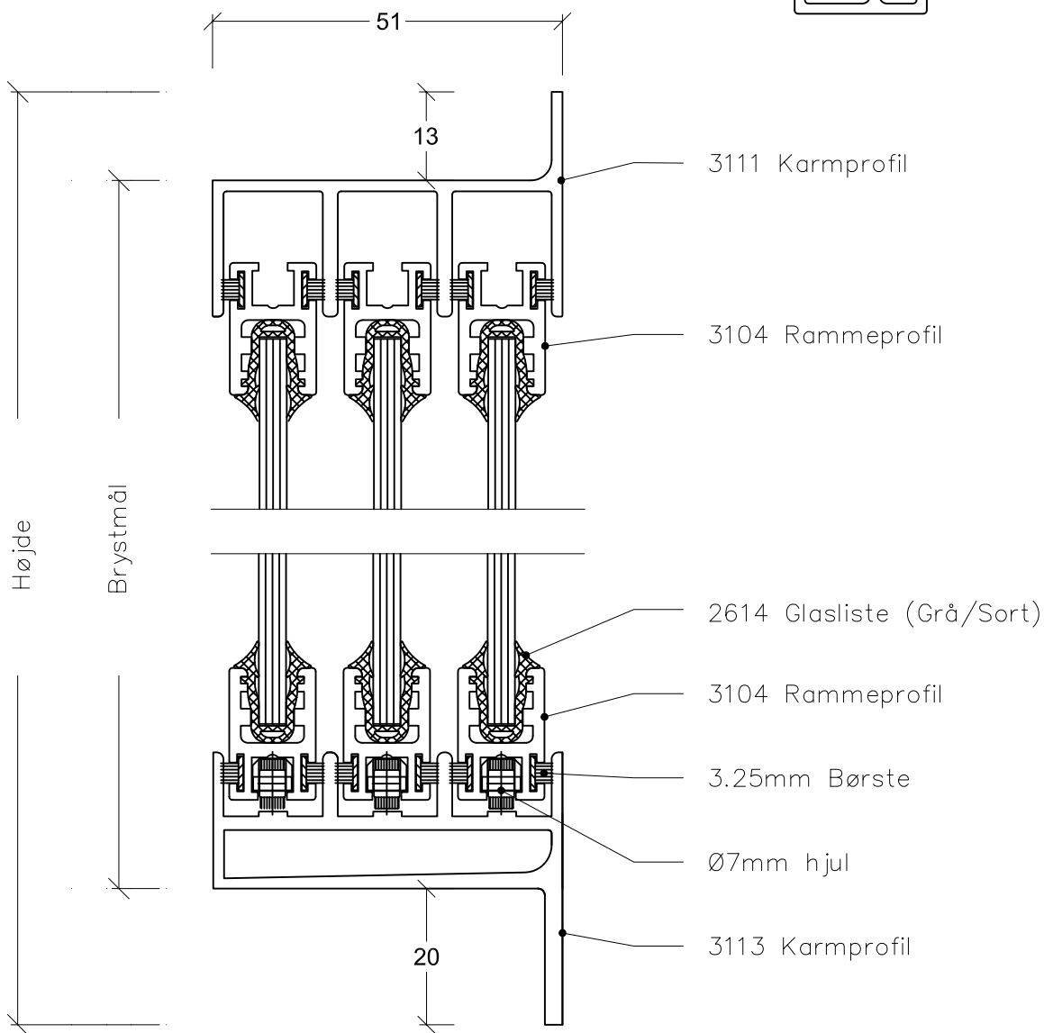
LODRET SNIT 1:1
