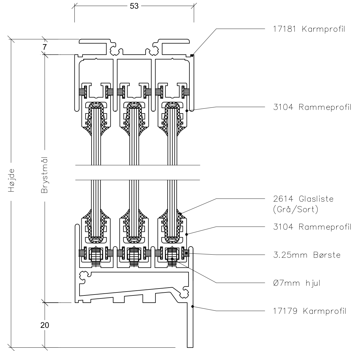
LODRET SNIT 1:1
