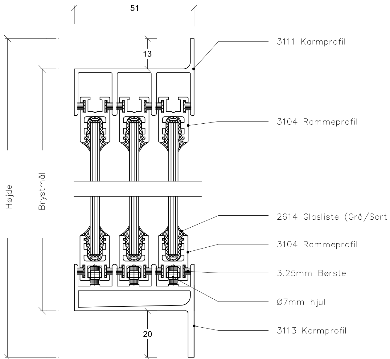
LODRET SNIT 1:1
