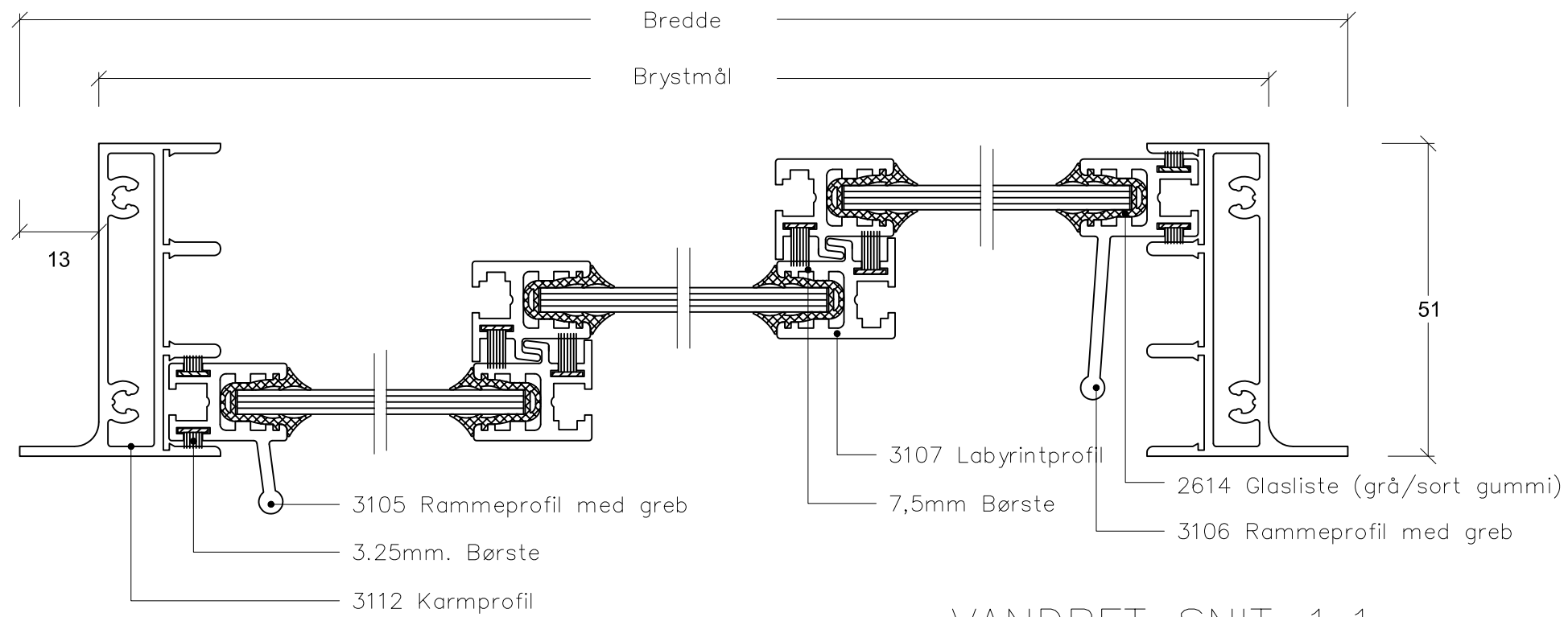
VANDRET SNIT 1:1
